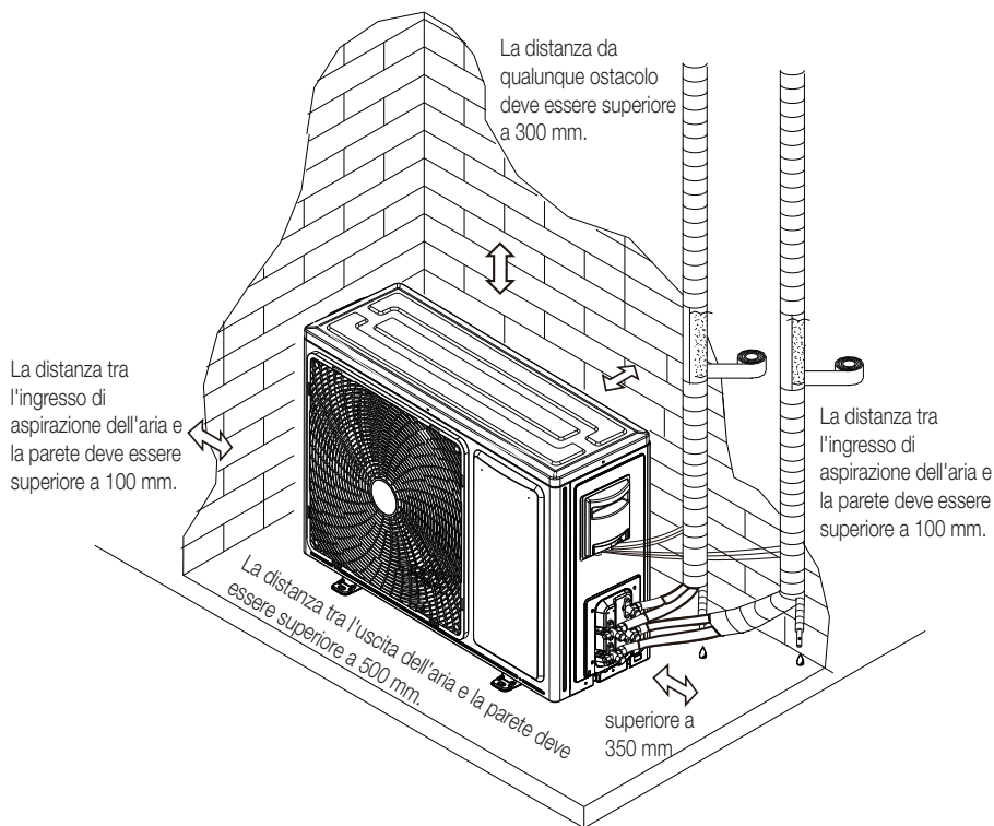
Unità esterna
